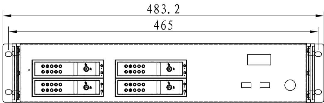
P向视图
