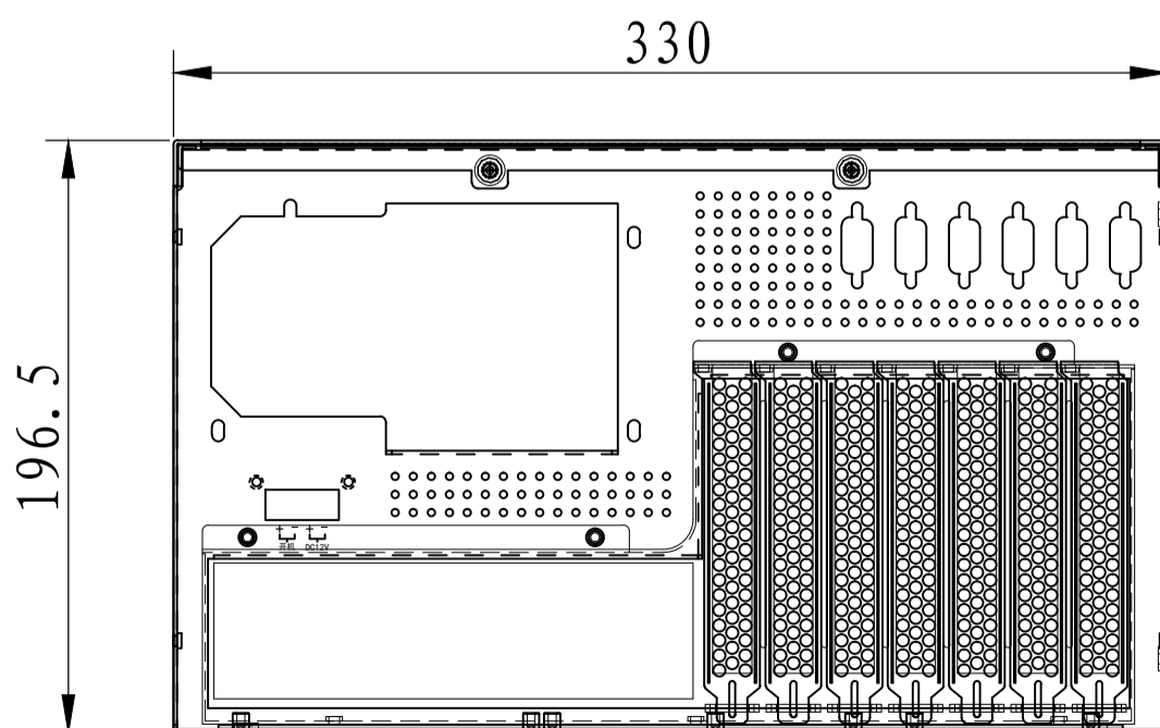
P向视图
