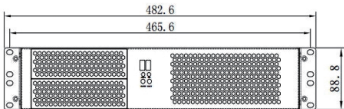
P向视图
