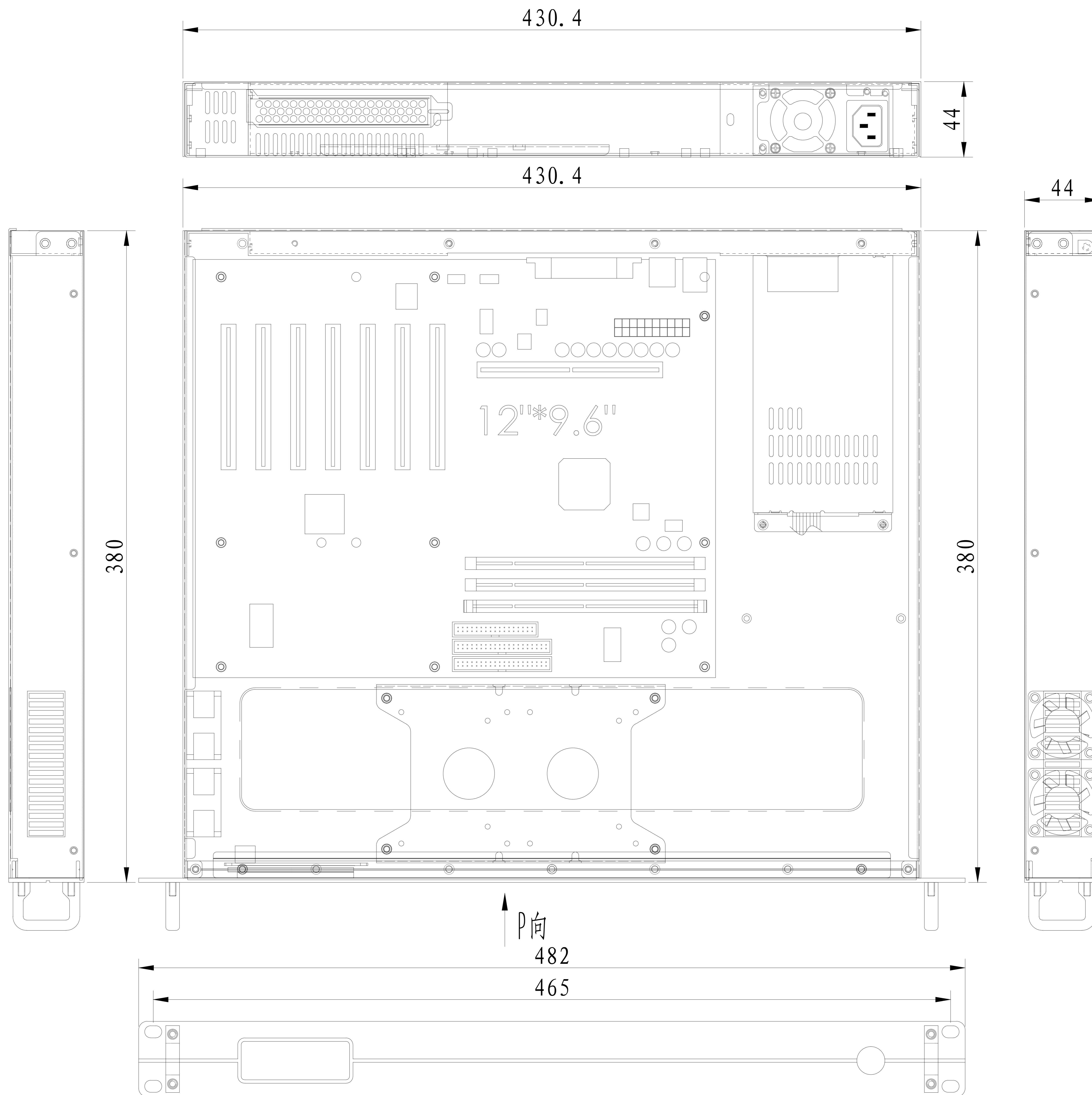
P向视图
